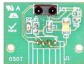
IRDA SENSE
